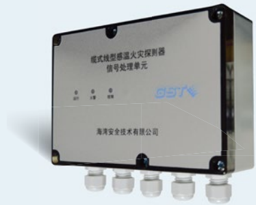
JTW-LD-GST85B/GST85A/GST105B 信号处理单元
